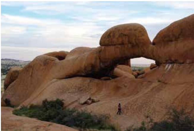
ナミビア白亜紀の風化した花崗岩
